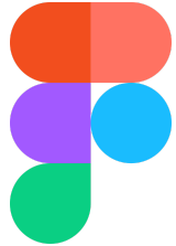
Figma
