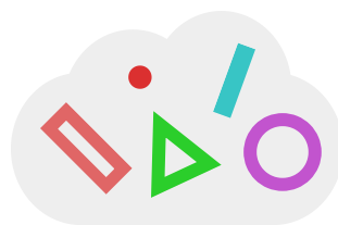
Figma API
