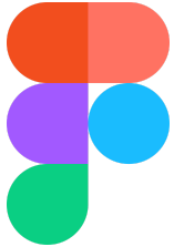
Figma
