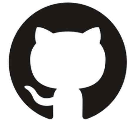
GitHub Codespaces
