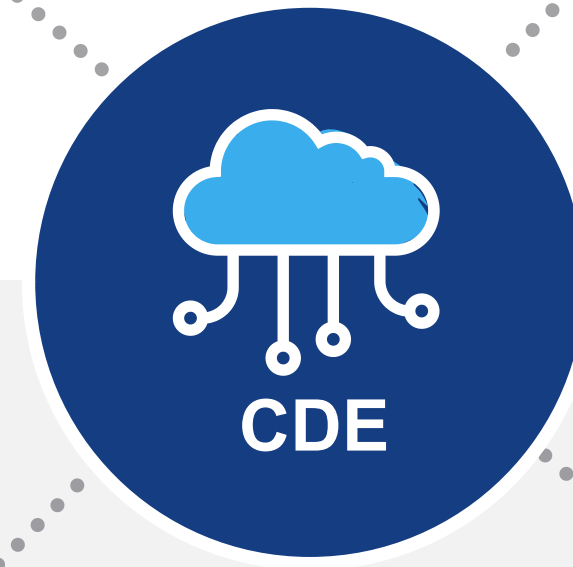
GitHub Codespaces
